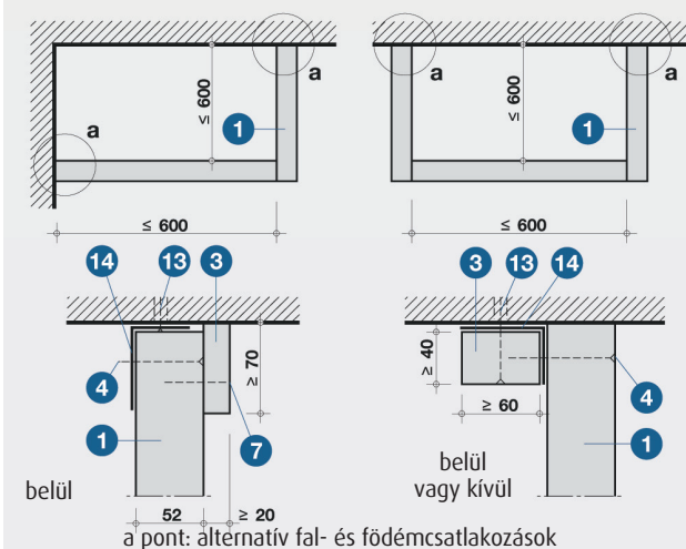
D részlet – két- és háromoldalas kivitel
