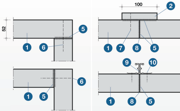
A részlet – sarokcsatlakozás
